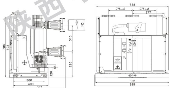
BGH型手车式外形及安装尺寸 (相间距210MM)
