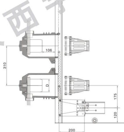
BGH-12P手车式断路器与800MM宽中置柜配合尺寸
