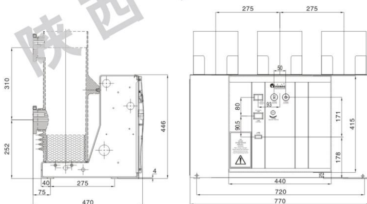
BGH型固定式外形及安装尺寸 (相间距210MM)
