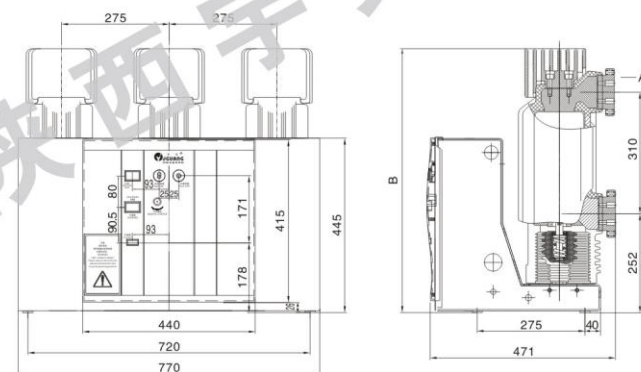
BGH型固定式外形及安装尺寸 (相间距210MM)
